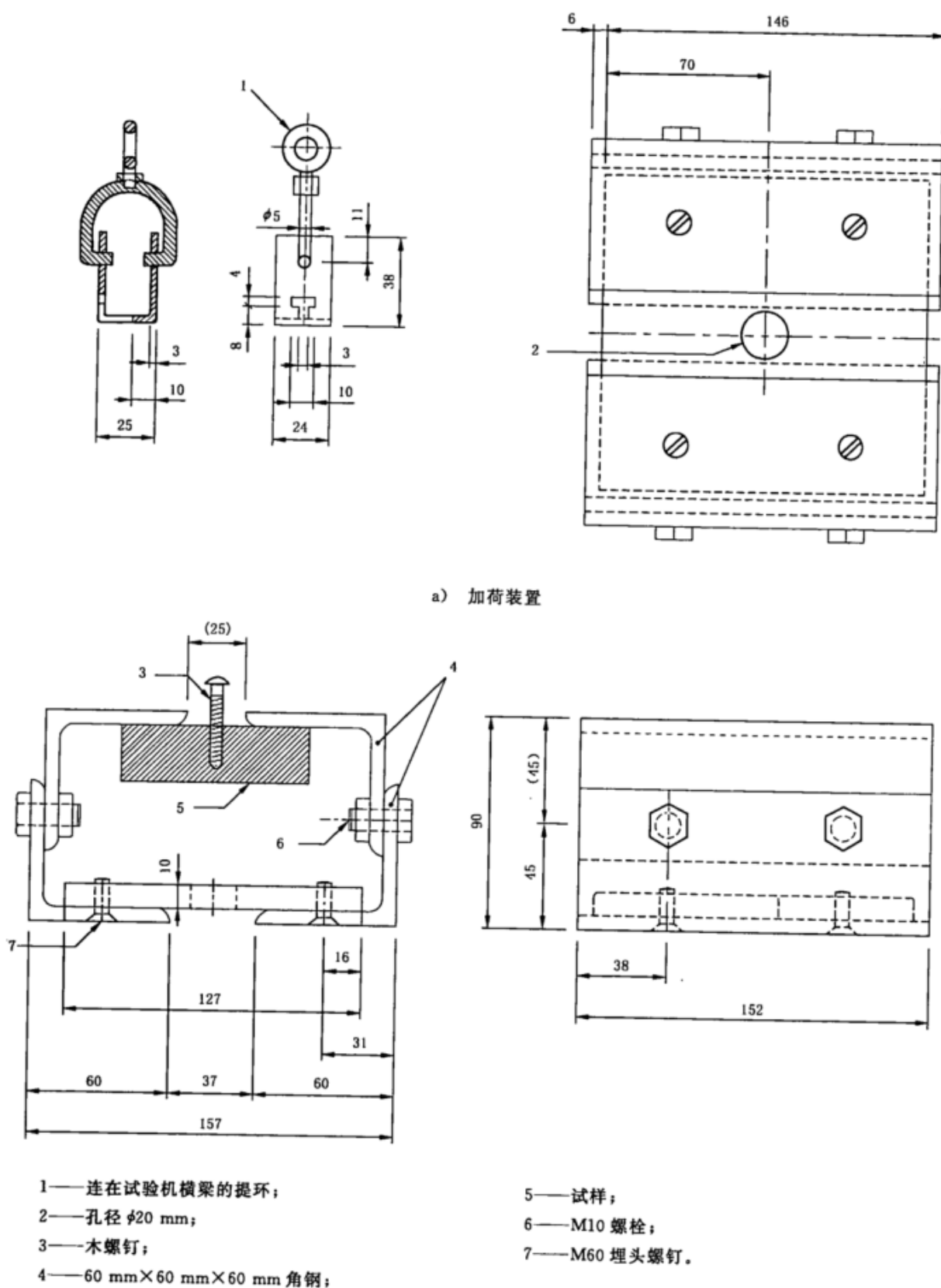
图 A.1 螺钉拔出试验的试样固定夹具和加荷夹具
